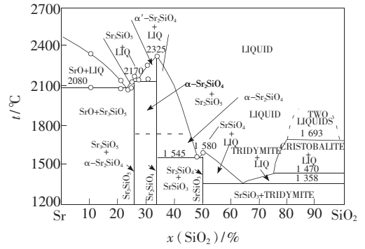
图 2 SrO-SiO 2 相图 [21]
