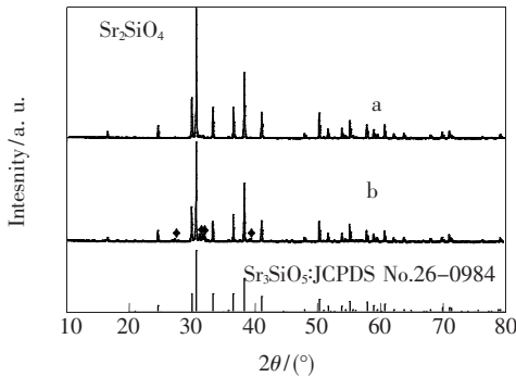
图 1 名义组成为 Sr 2.980 Si 0.980 Al 0.020 O 5 :0.020Ce 3+ 荧光粉的 XRD 谱。(a) 非均相沉淀法制备;(b) 高温固相反应法制备。
